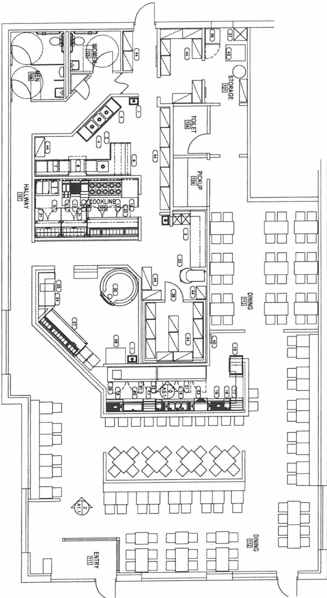
1 LAYOUT A1.0 SCALE: 1/4" = 1'-0" N →
